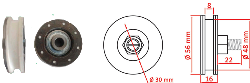
SHPE 996 - Roldana para porta modelo At120 56 mm original
