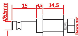
SHPE 525 - Pino concêntrico 3/8"
