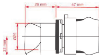
SHPE 341 - Chave seletora 2 posições
