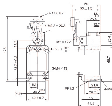
• Corpo metálico • Haste não ajustável • Roldana metálica Ø 17,5 mm
