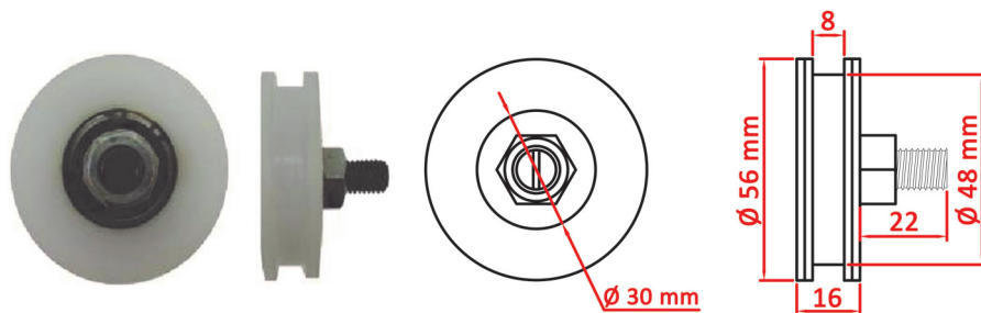
SHPE 997 - Roldana para porta similar At120 56 mm
