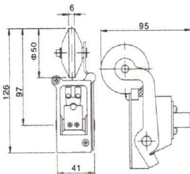
SHPE 710 - Limite switch NF
