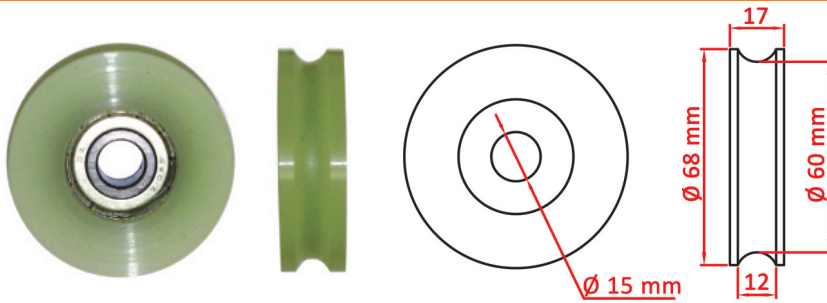
SHPE 986 - Para porta de cabina 68 mm
