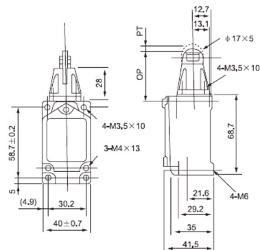
• Corpo metálico • Roldana metálica Ø 17 mm
