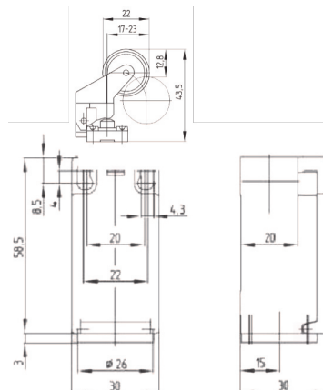
SHPE 716 - Limite ZK4 236 11ZP 18843002
