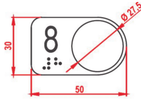
SHPE 222 - Pastilha braille inox 50 x 30 mm
