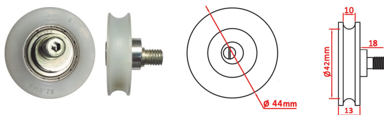
SHPE 1026 - Roldana inferior 44 mm completa
