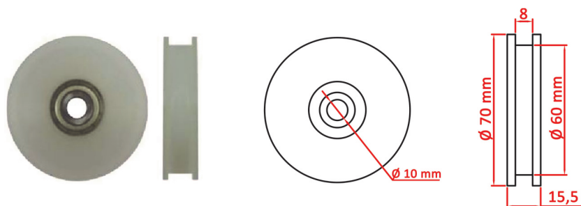
SHPE 1000 - Roldana de porta 70 mm
