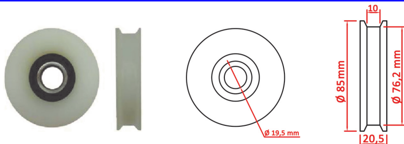
SHPE 1001 - Roldana de porta 85 mm
