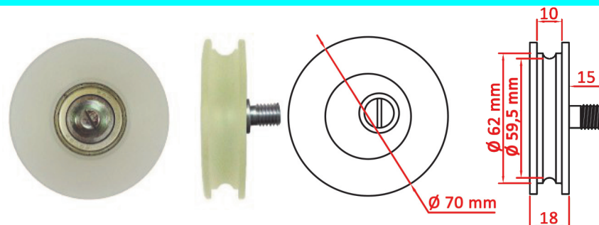
SHPE 989 - Para suspensão de porta de cabina
