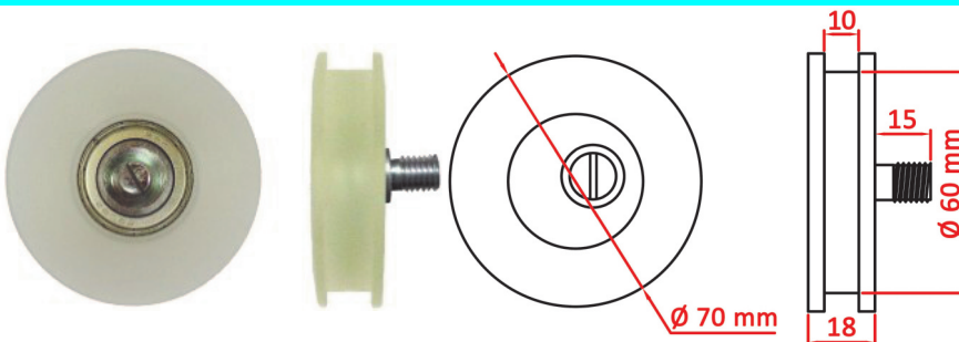
SHPE 988 - Para suspensão de porta de cabina 70 mm canal reto com eixo
