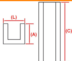
SHPE 452 - Para cabina com abas (L:33xA:23xC:117 mm)
