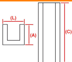
SHPE 454 - Para cabina com abas (L:21xA:33xC:198 mm)
