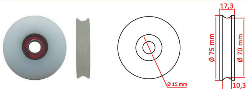
SHPE 1022 - Roldana para porta de cabina 75 mm
