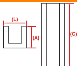
SHPE 453 - Para cabina com abas (L:21xA:33xC:149 mm)
