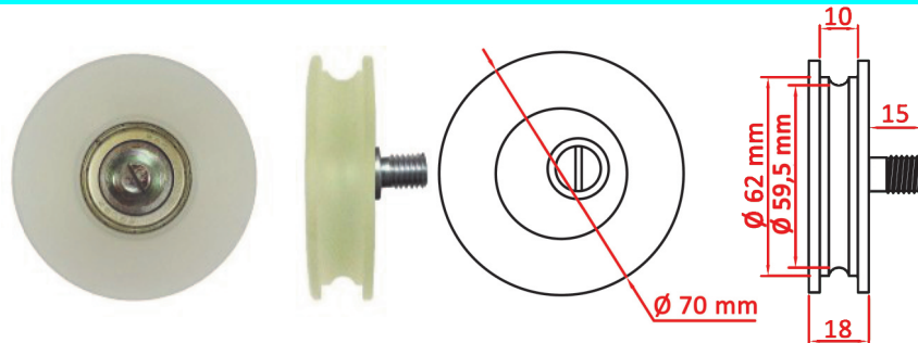
SHPE 989 - Para suspensão de porta de cabina 70 mm com eixo
