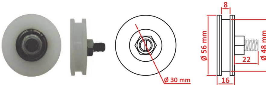
SHPE 997 - Roldana para porta similar At120 56 mm
